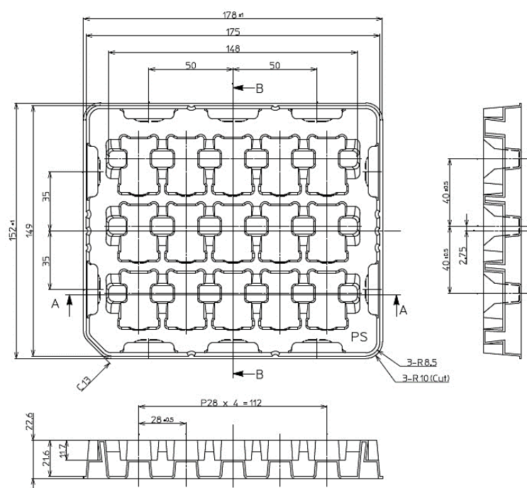
A-A section
